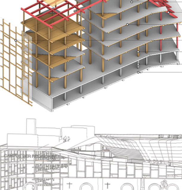
Konstruktionsprinzip und Tragwerk Gebäude
