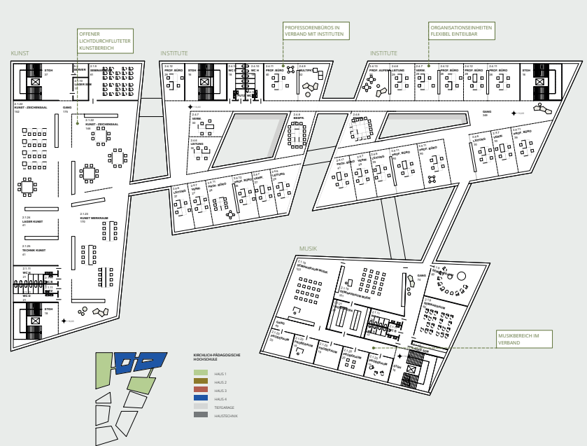
OBERGESCHOSS 5 M 1:250
