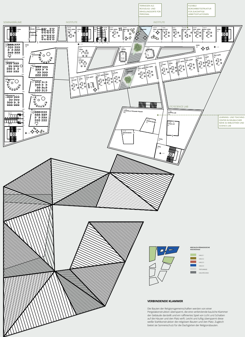
OBERGESCHOSS 3 M 1:250
