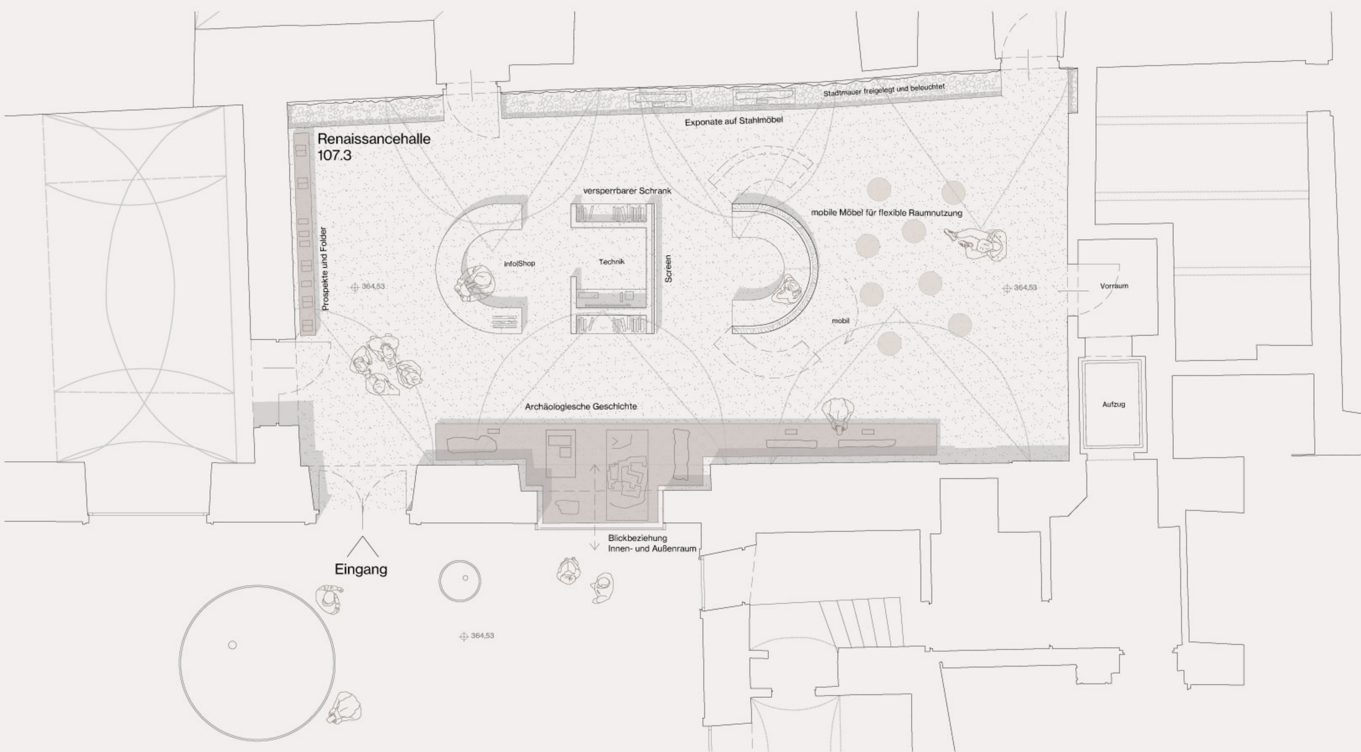
Grundriss Karlstrakt 1:50
