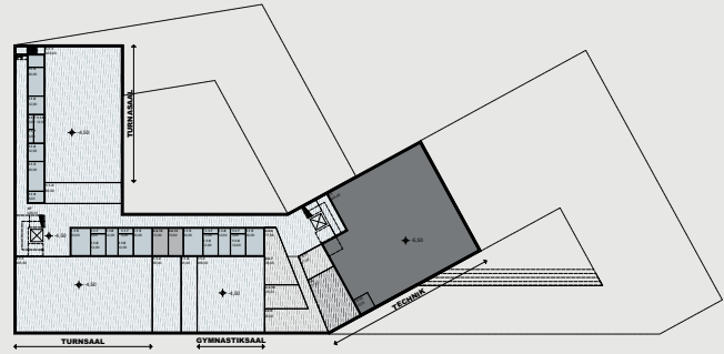
GRUNDRISS KG | 1:500
