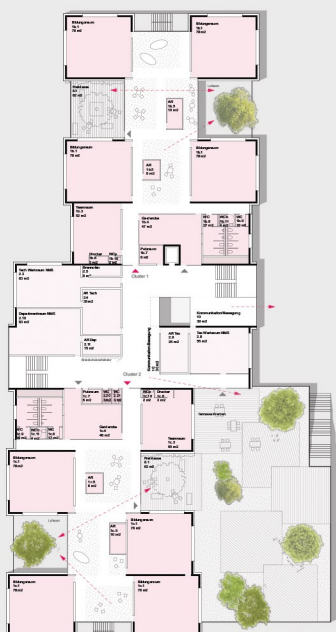
1. Obergeschoß 1:250
