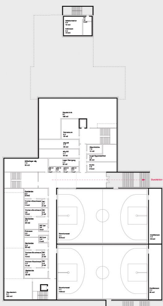
Untergeschoß 1:250
