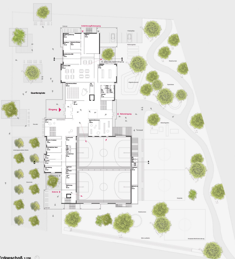
Erdgeschoß 1:250
